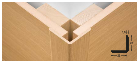
Winkleleiste WKL 28/28 Länge 2380 mm
